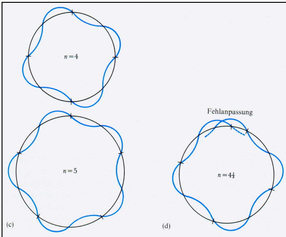
Abb. 11: Elektronenwellen in einer Bohrschen Umlaufbahn
