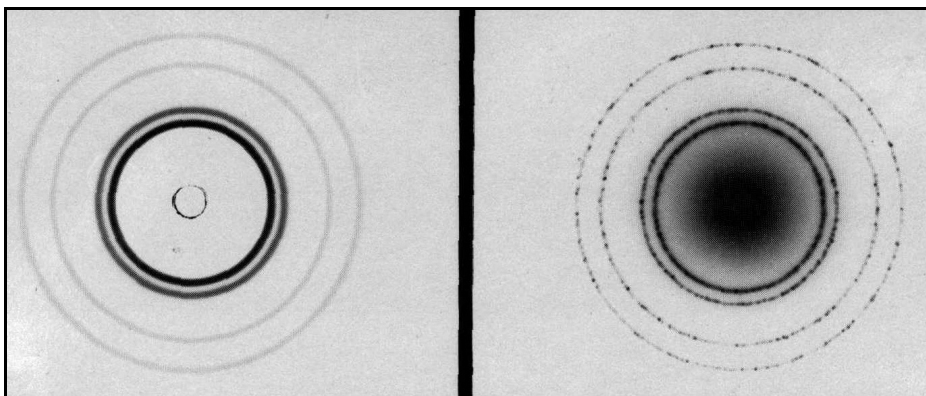
Abb. 12: Beugung von Röntgenstrahlen durch eine Alu-Folie (links) und Elektronenstrahlen (rechts), invertiertes Bild.
