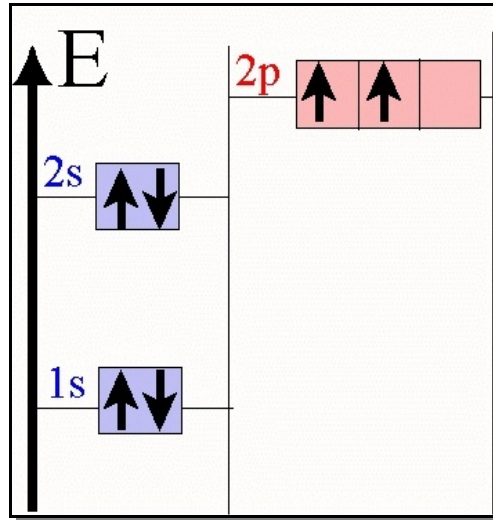
Abb. 21: Elektronen- konfiguration des C-Atoms
