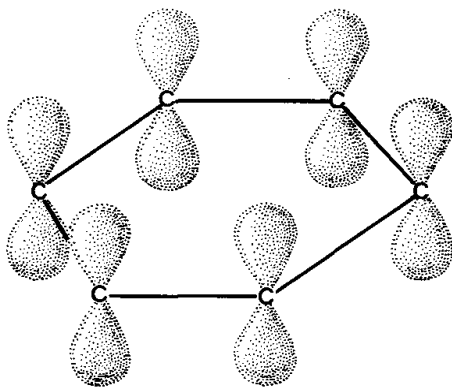
Abb. 7/1. Anordnung der p-Orbitale im C-Gerüst von Benzol.
