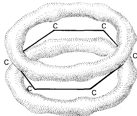
Abb. 7/2. Überlappung der p-Orbitale zu delokalisierten π-Bindungen im C-Gerüst von Benzol.
