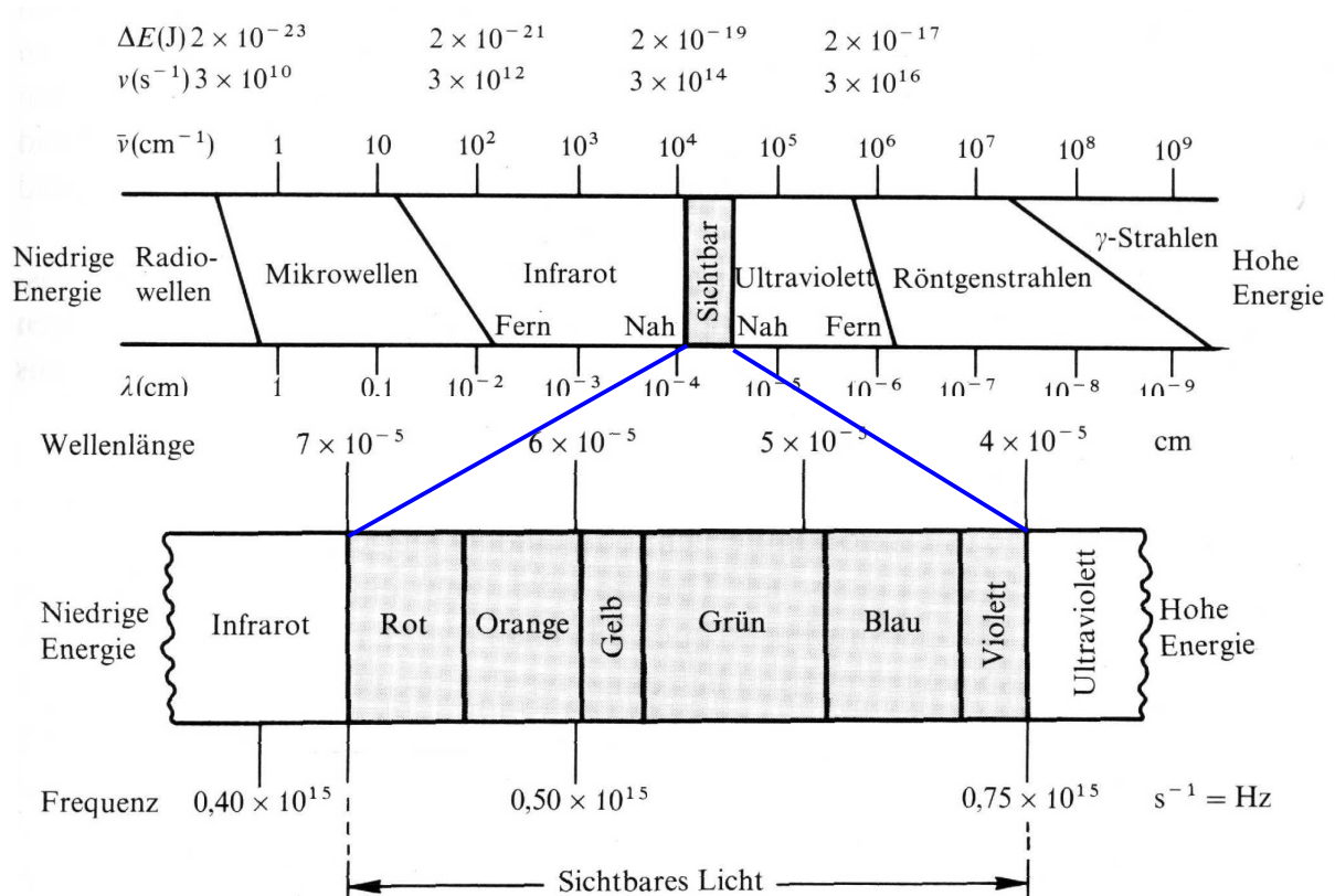
Abb.3.: Spektrum der elektromagnetischen Strahlung mit logarithmischer Skala
