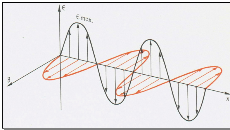
Abb.2.: Momentbild einer in x-Richtung sich ausbreitenden elek- tromagnetischen Welle; E: elektr. Feldstärke, B: magnetische Feldstärke
