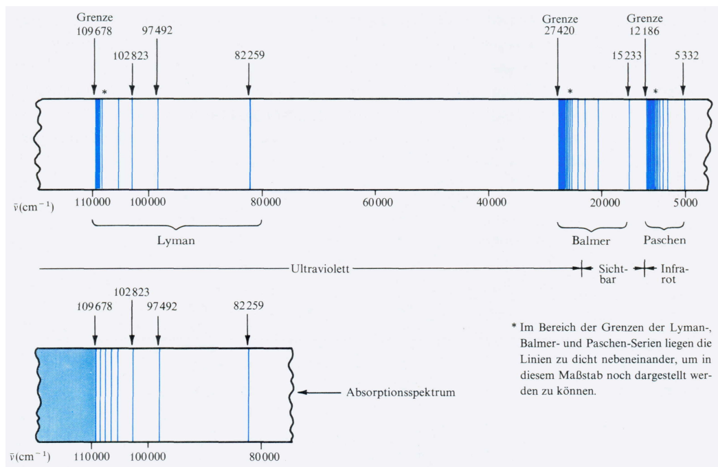
Abb. 5: Emissions- und Absorptionsspektrum des Wasserstoffs
