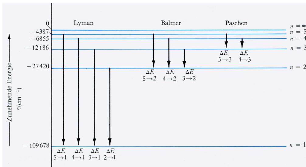
Abb. 6: Energieniveaudiagramm des H-Atoms
