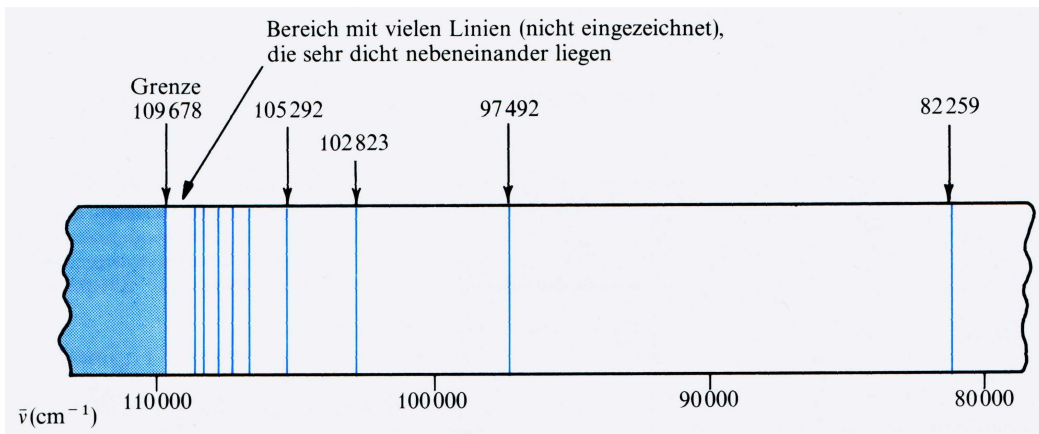
Abb. 5-1: Emissionsspektrum des Wasserstoffs
